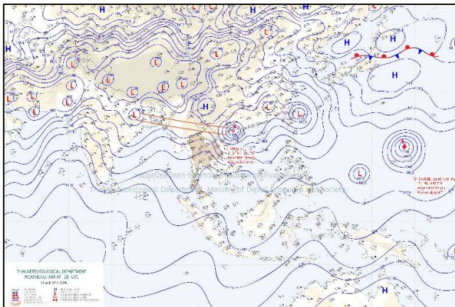
แผนที่อากาศ วันที่ ๒๒ ส.ค. ๒๕๖๙ เวลา ๐๑.๐๐ น.
