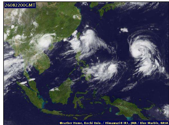
ภาพถ่ายดาวเทียม วันที่ ๒๒ ส.ค. ๒๕๖๙ เวลา ๐๗.๐๐ น.
